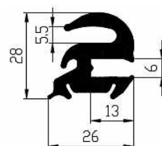
Order No. Mixture Nozzle VP6117 EPDM 70 BXK VP6199 EPDM 50 BXK VP6200 EPDM 60 BXK
